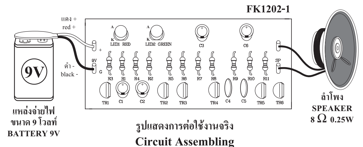
รูปแสดงวงจรเสียงไซเรนพร้อมไฟกะพริบ LED 2 ดวง POLICE SIREN WITH LED FLASHER 2 LED
